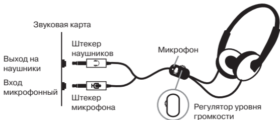
Рис. 1. Схема подключения
